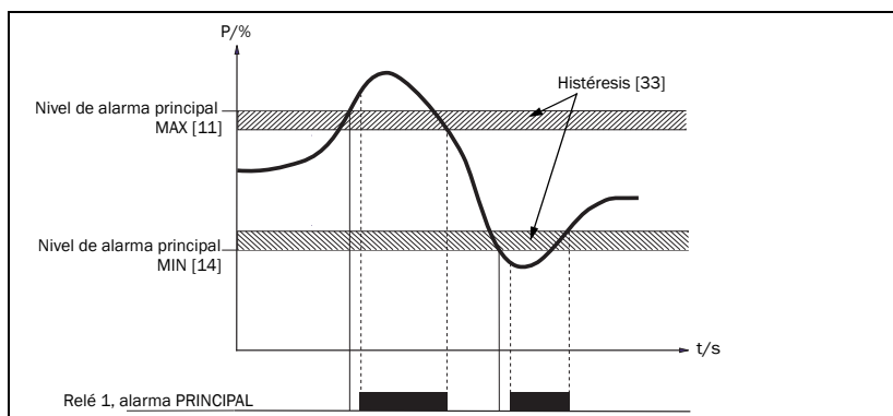
Figura 10 Histéresis.
