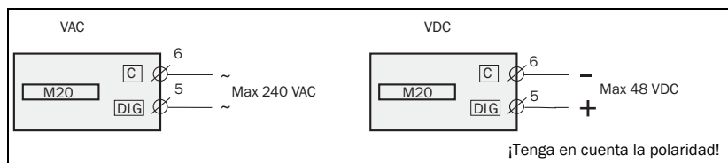
Figura 3 Ejemplo de cableado para entrada digital.
